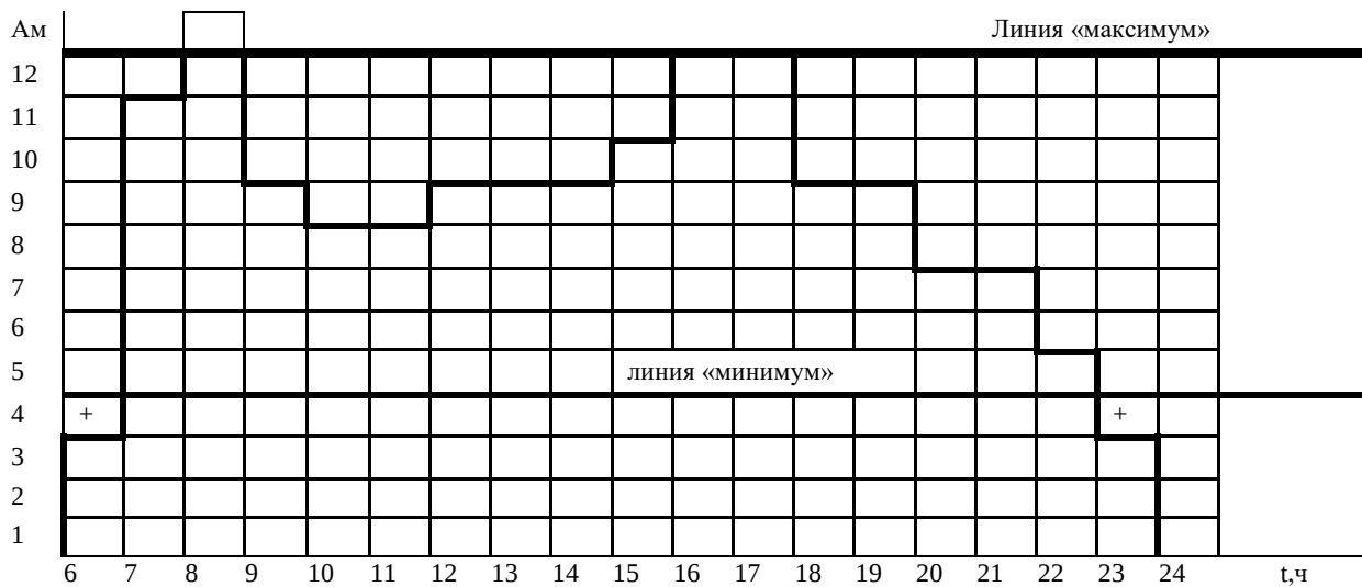
Рисунок 3.1 - Диаграмма «максимум»
